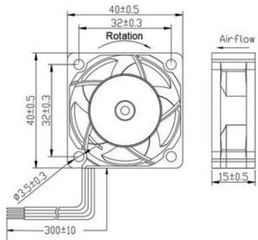
产品结构尺寸
